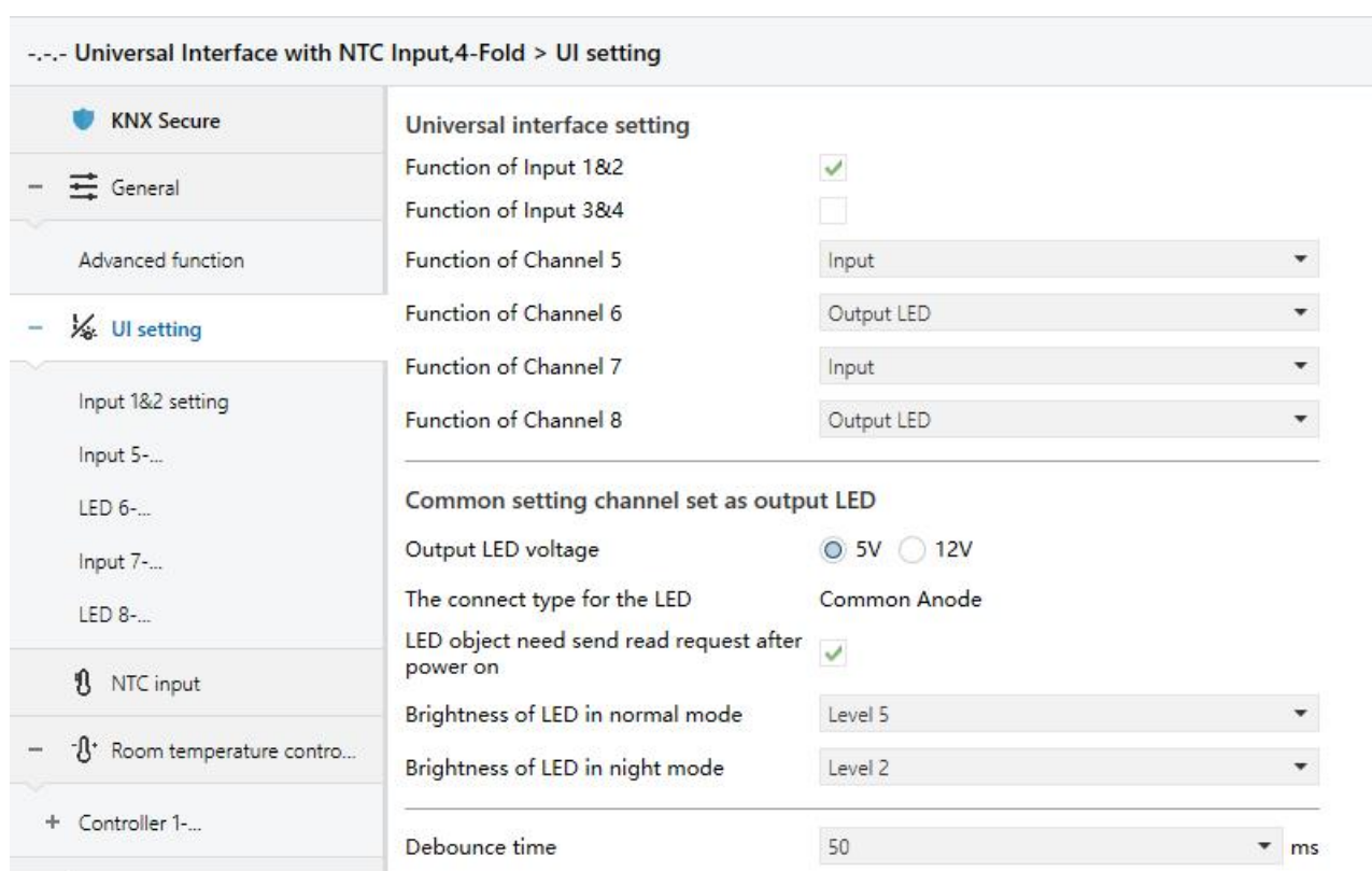
Fig.4.6 parameter window “UI setting”
