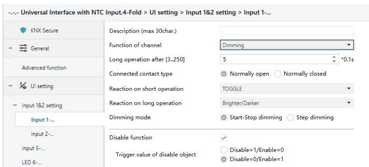
Fig.4.6.2.2 parameter window “Input x- Dimming”
