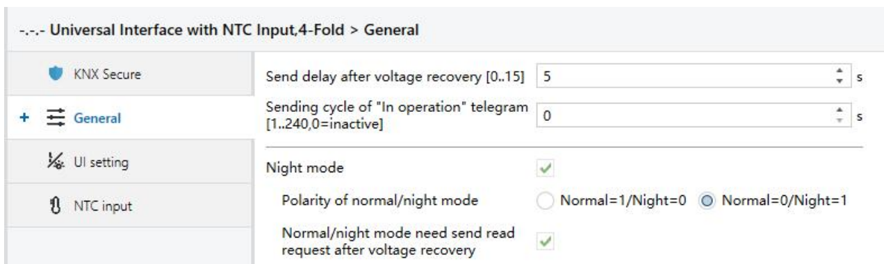
Fig.4.2.1 “General setting” parameter window
