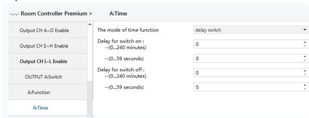
Fig. 5.17 parameter window “X: Time-Delay switch”
