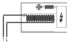
2-pipe fan coil
