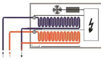
3-pipe fan coil
