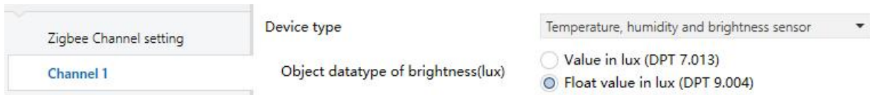
Fig.5.3.2 "Channel setting" Parameter window
